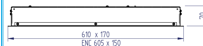
Modèle pour encastrement dans faux-plafond
